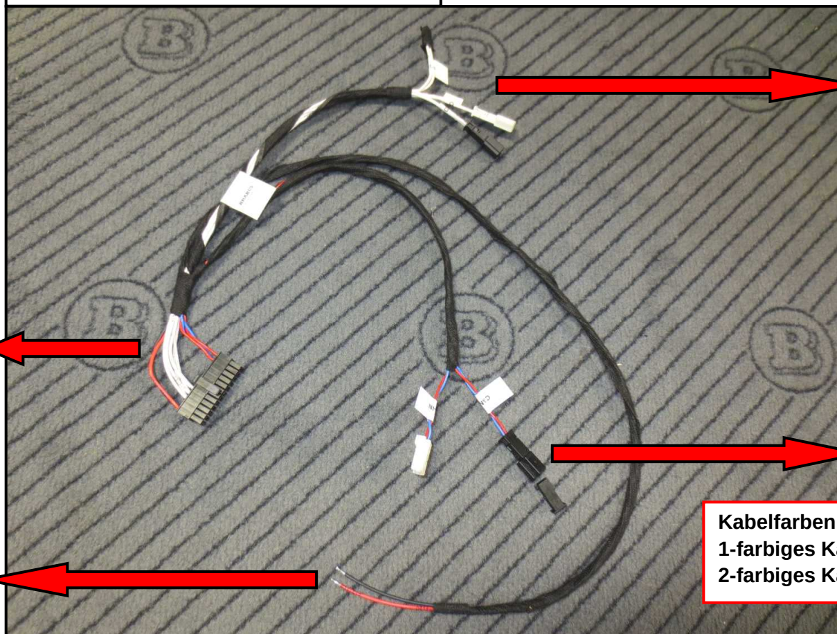
Innenraum-Kabelsatz 176-700-00-K
