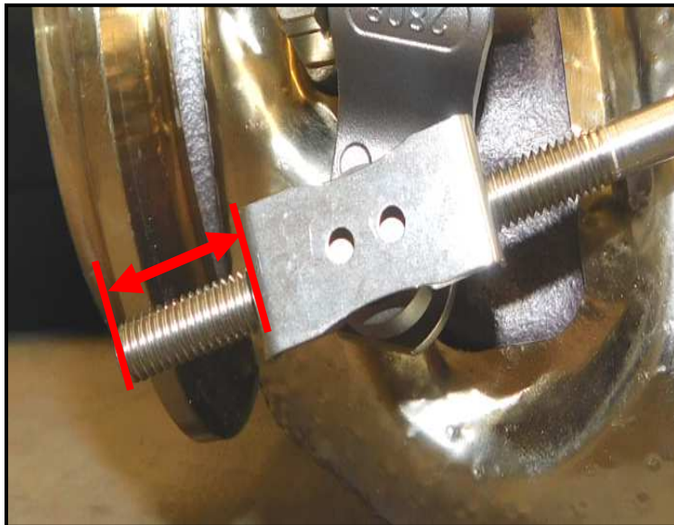
Die gefräste Fläche ist Merkmal des in Fahrtrichtung linken Turboladers
